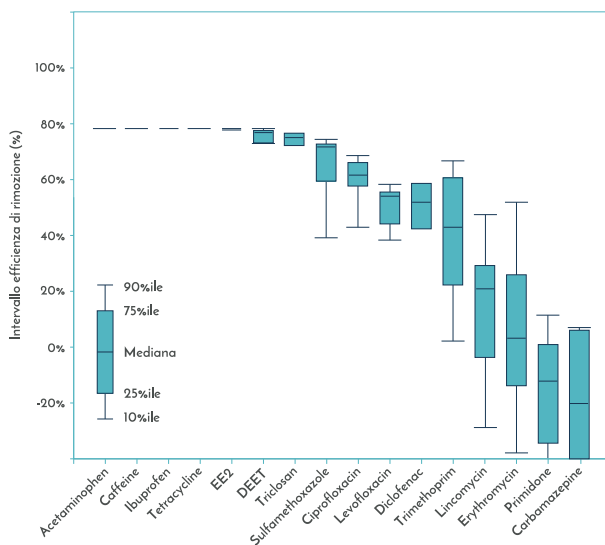
Fig. 2.2 – Efficienza di rimozione di alcuni microinquinanti in sistemi MBR (Yang et al. , 2011, come modificata da Rodriguez-Narvaez et al. , 2017)
