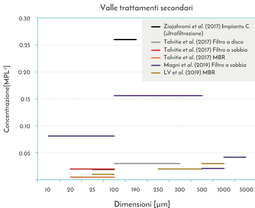
Fig. 3.10 – Distribuzione per dimensione e concentrazione delle microplastiche a valle di trattamenti terziari (modificato da: Baruta, 2019).
