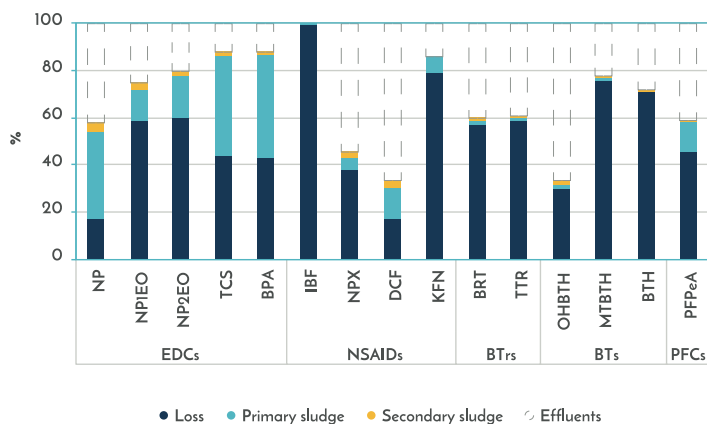
Fig. 2.9 - Comportamento di alcuni composti in impianto di depurazione (distruttori endocrini EDC, antiinfiammatori non steroidei NSAID, benzotriazoli BTr, benzotiazoli BT, composti perfluorurati PFC) (da Stasinakis et al. , 2013, modificata).
