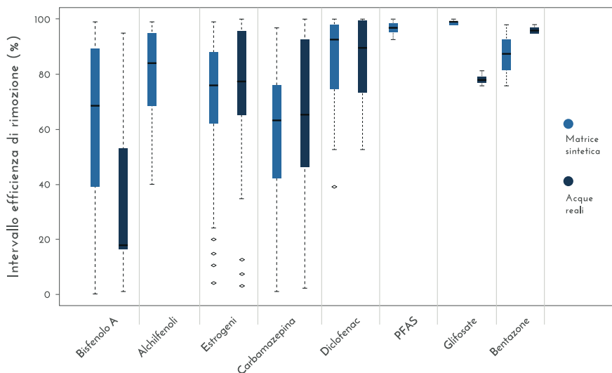
Fig. 2.5 - Intervallo di efficienza di rimozione dei MIE per separazione a membrana riportate nelle risorse bibliografiche esaminate in funzione della matrice dell'acqua utilizzata negli esperimenti.
