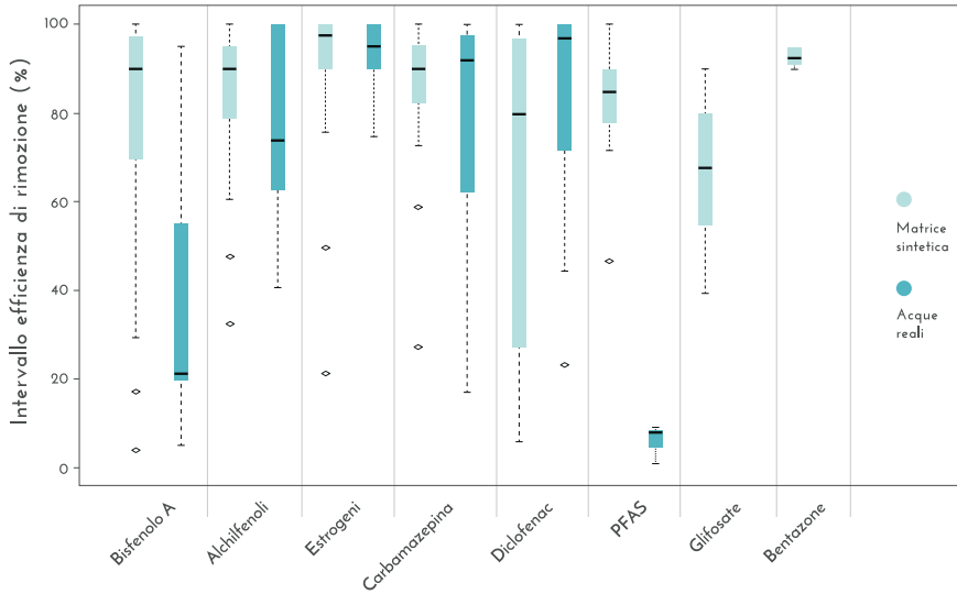
Fig. 2.6 – Intervallo di efficienza di rimozione dei MIE per ossidazione con ozono o AOP riportate nelle risorse bibliografiche esaminate in funzione della matrice dell'acqua utilizzata negli esperimenti.
