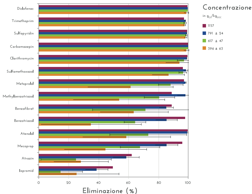
Fig. 2.11 – Rimozione percentuale di una serie di microinquinanti organici con diversi dosaggi di ozono (Schaerer, 2012).
