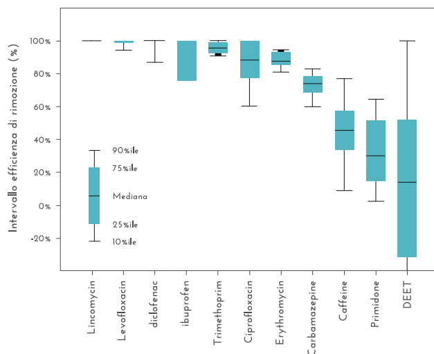
Fig. 2.7 – Efficienza di rimozione di alcuni microinquinanti in fase terziaria mediante carbone attivo (Yang et al. , 2011, come modificata da Rodriguez-Narvaez et al. , 2017).
