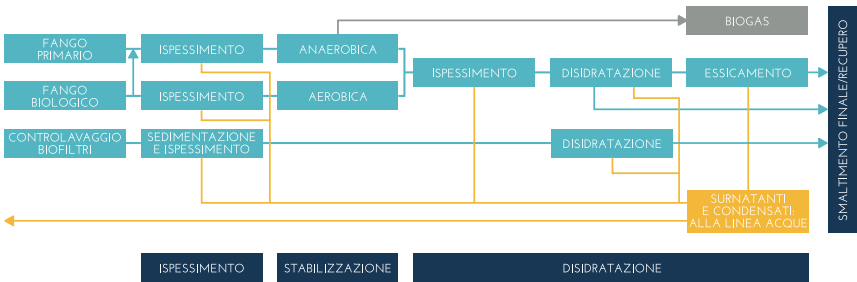
Fig. 2.8 - Schema delle fasi ed operazioni presenti in linea fanghi.
